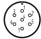
七芯航插
